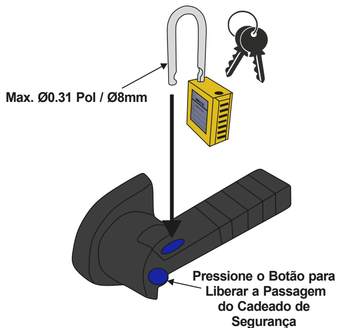
Acessórios (2) Manopla Redonda
