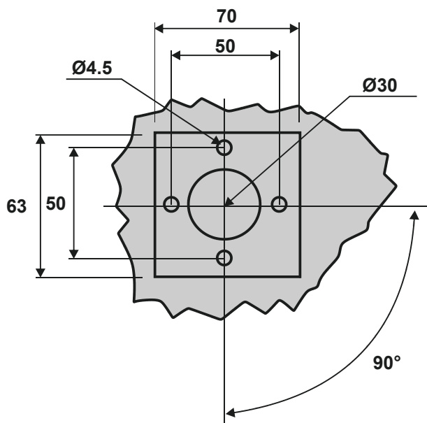
Acessórios (1) Manopla Quadrada
